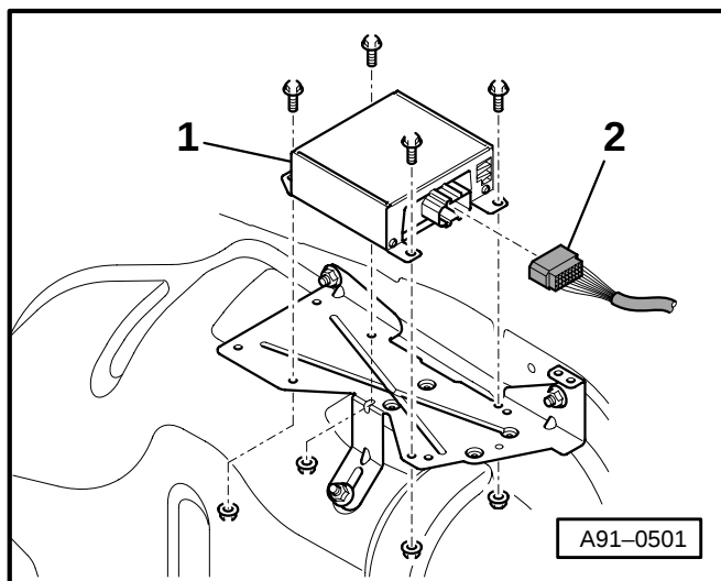
Fig. 4 Amplifier - R12
